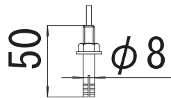
アンカーボルト C-850
